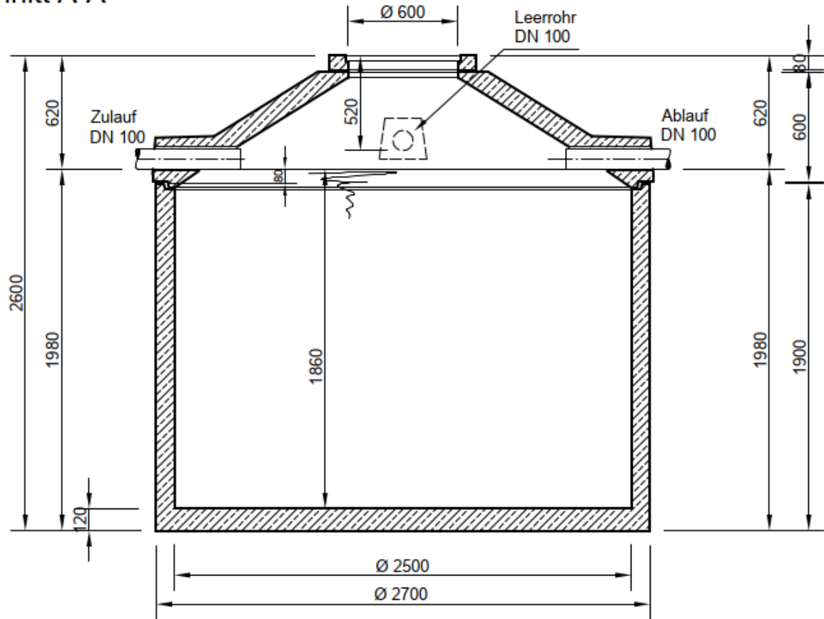
Schnitt A-A
