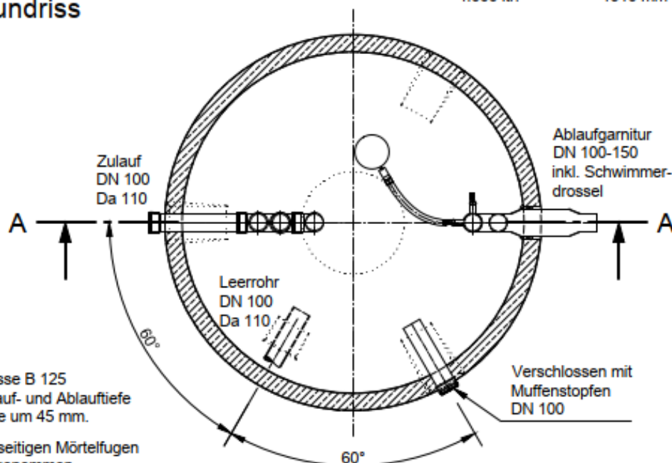
Grundriss
