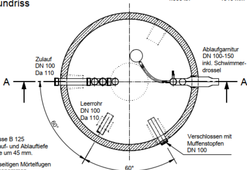
Grundriss
