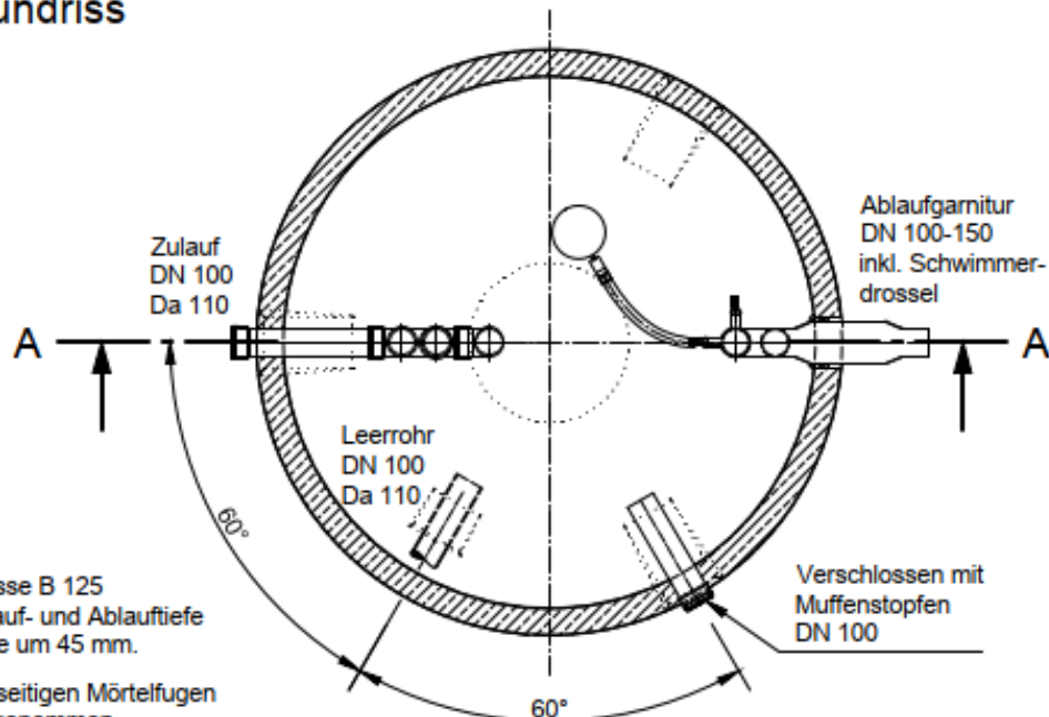
Grundriss
