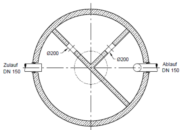
GRUNDRISS
