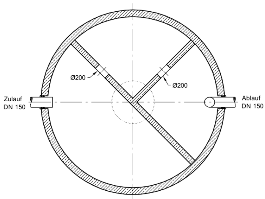
GRUNDRISS
