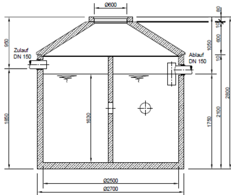
SNITT
