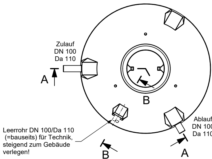
Draufsicht
