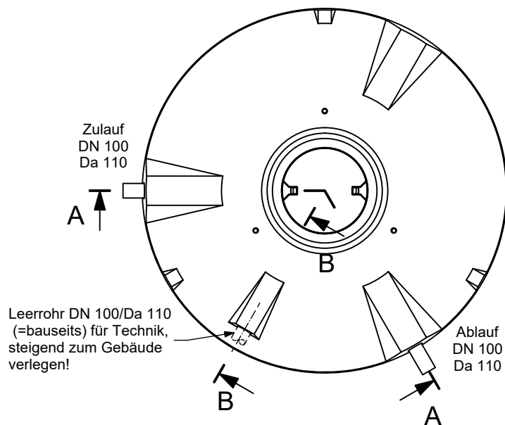
Draufsicht
