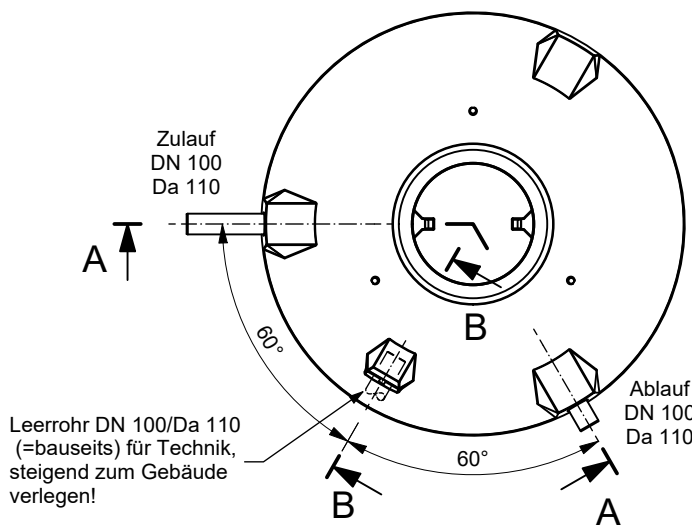
Draufsicht
